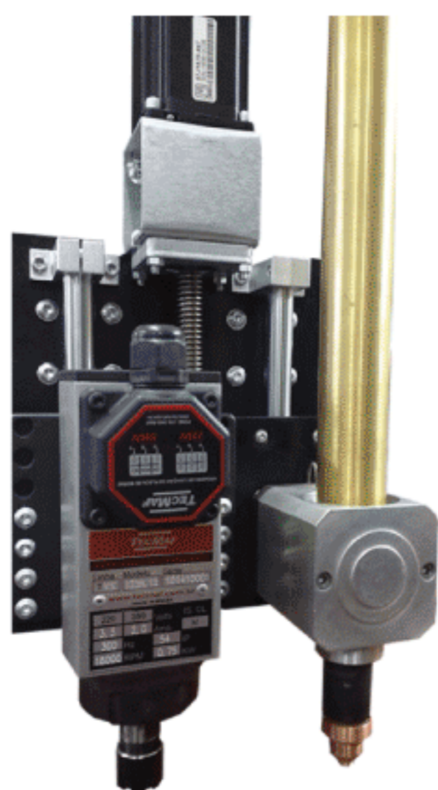
Cabeçote Híbrido
